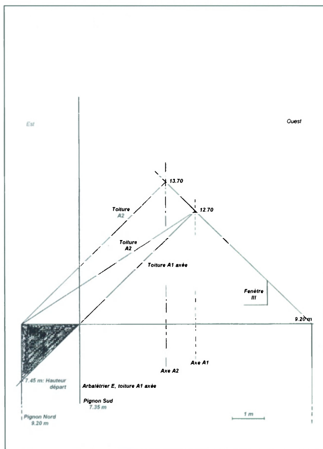
Fig. 33. - Hypothèses de reconstitution d'une toiture axée sur A1. Dessin de l'auteur.
