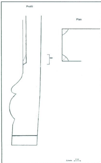
Fig. 29. - Structure A, façade nord, intérieur : profil du piedroit ouest de la cheminée. Dessin de l'auteur.
