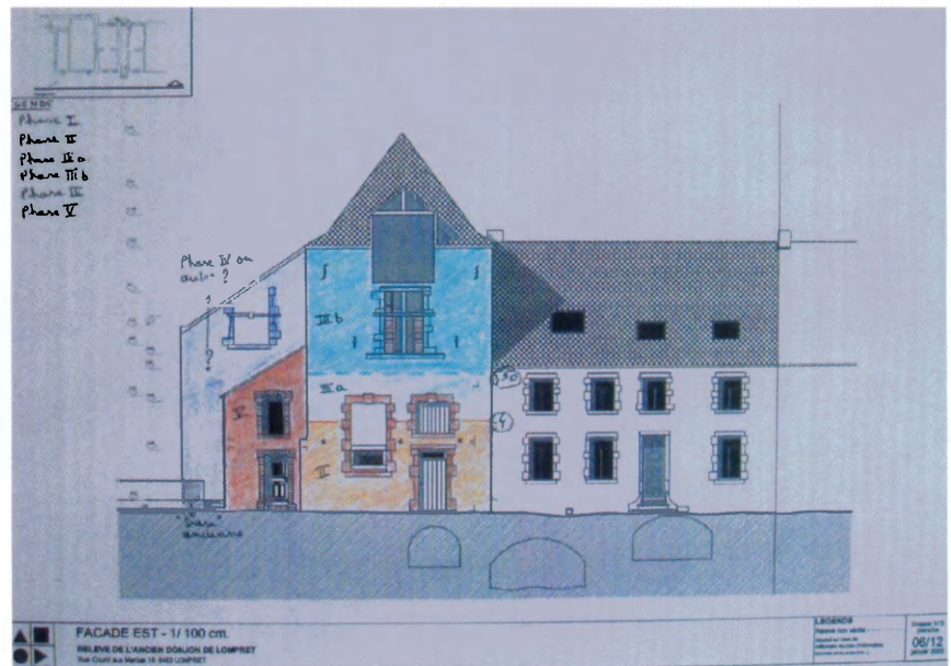
Fig. 19. - Relevé d'ensemble du mur est des structure A, B et de l'annexe sud-est. Architecte Jean de Salle, Dossier d'étude préliminaire à la restauration du donjon de Lompret, fascicule de plans n°3, Cooparch - R.U. scrl avec le soutien de la Fondation Wartoise, 2006.
