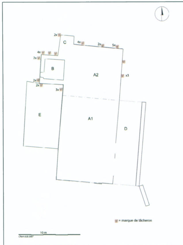
Fig. 22. - Plan d'ensemble du bâtiment avec répartition des marques sur les niveaux supérieurs (deuxième niveau et combles). Relevé de l'auteur avec l'aide du CRéA.
