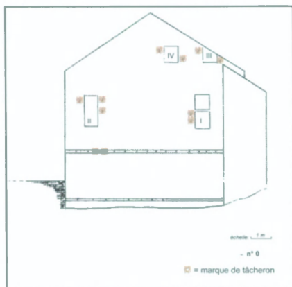
Fig. 7. - Structure A, façade nord : schéma d'élévation avec distribution des marques de tâcheron. Dessin de l'auteur.
