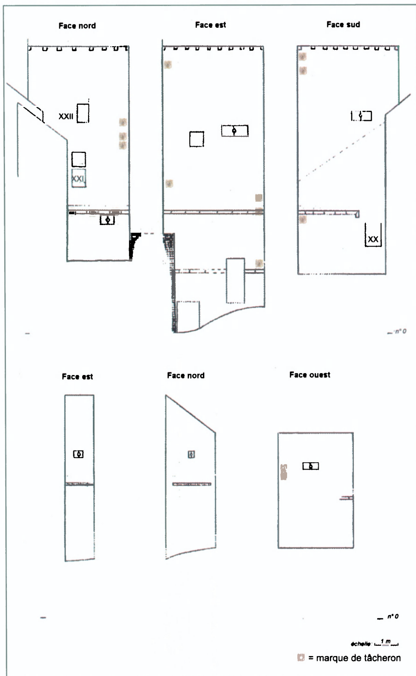
Fig. 8. - Tour B (haut) et « tourelle » C (bas) : schémas d'élévation avec distribution des marques de tâcheron. Dessin de l'auteur.
