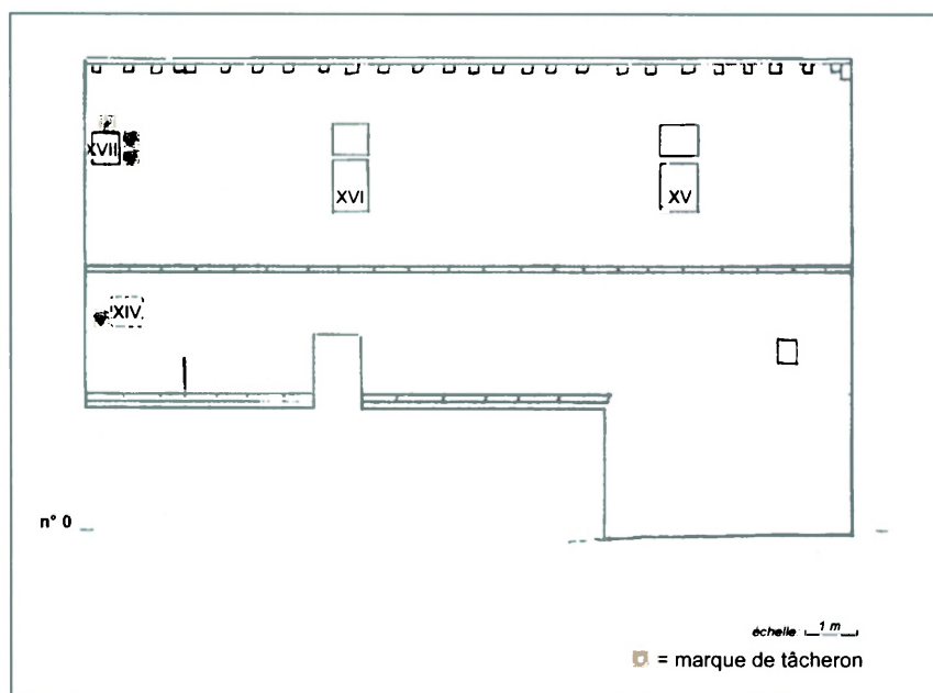
Fig. 19. - Structure A, façade ouest : schéma d'élévation avec distribution des marques de tâcheron. Dessin de l'auteur.
