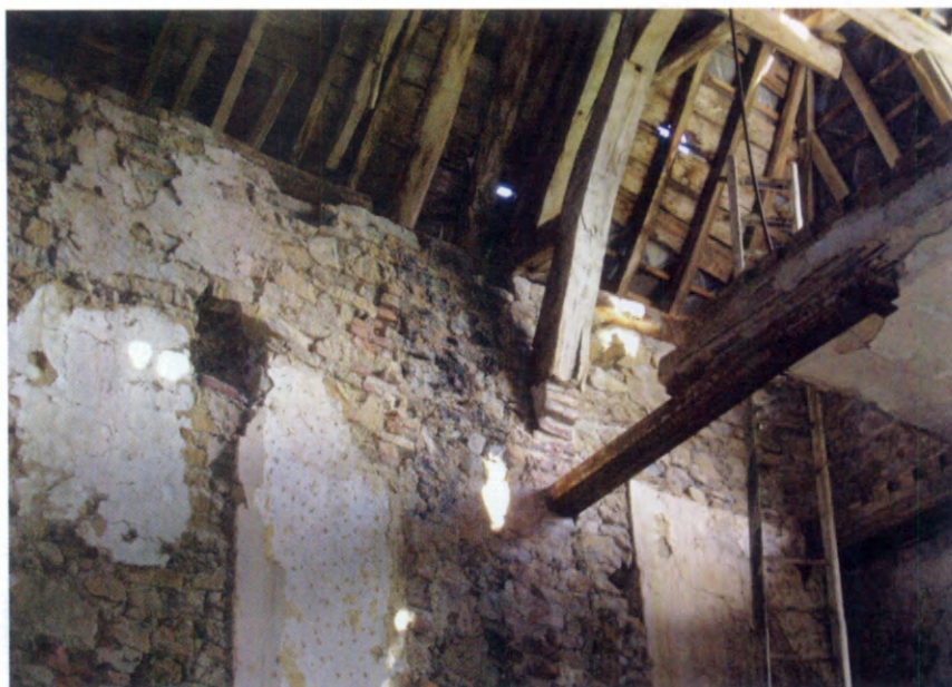
Fig. 33. - Vue des anciens trous de poutres situés dans la partie supérieure du mur nord de la structure A, angle nord-est. © Clémence Mathieu, 2006.
