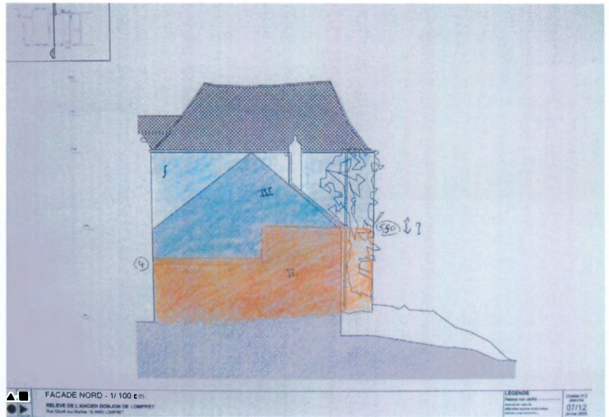
Fig. 17. - Relevé d'ensemble du mur nord de la structure A. Architecte Jean de Salle, Dossier d'étude préliminaire à la restauration du donjon de Lompret, fascicule de plans n°3, Cooparch - R.U. scrl avec le soutien de la Fondation Wartoise, 2006.
