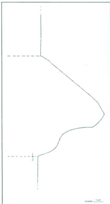
Fig. 11. - Structure A, façade nord : profil du larmier. Dessin de l'auteur.
