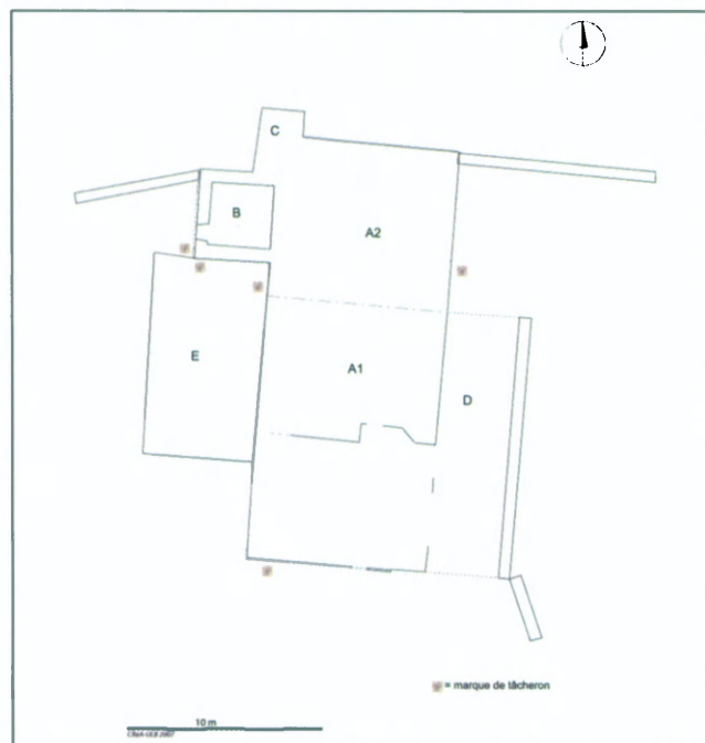
Fig. 21. - Plan d'ensemble du bâtiment avec répartition des marques au niveau du bel étage. Relevé de l'auteur avec l'aide du CRéA.
