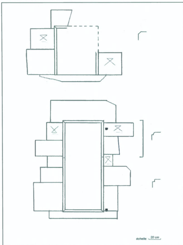
Fig. 20. - Structure A, façade nord : relevé de la fenêtre haute (II ; bas) et de la fenêtre coupée par la toiture actuelle (III ; haut). Dessin de l'auteur.
