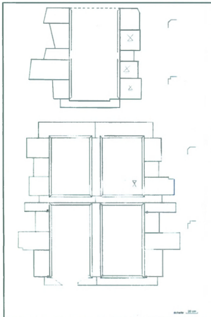
Fig. 17. - Structure A, façade est : relevé d'une fenêtre à croisée (VII ; bas) et d'une ancienne fenêtre à traverse (bûchée) (IX ; haut). Dessin de l'auteur.
