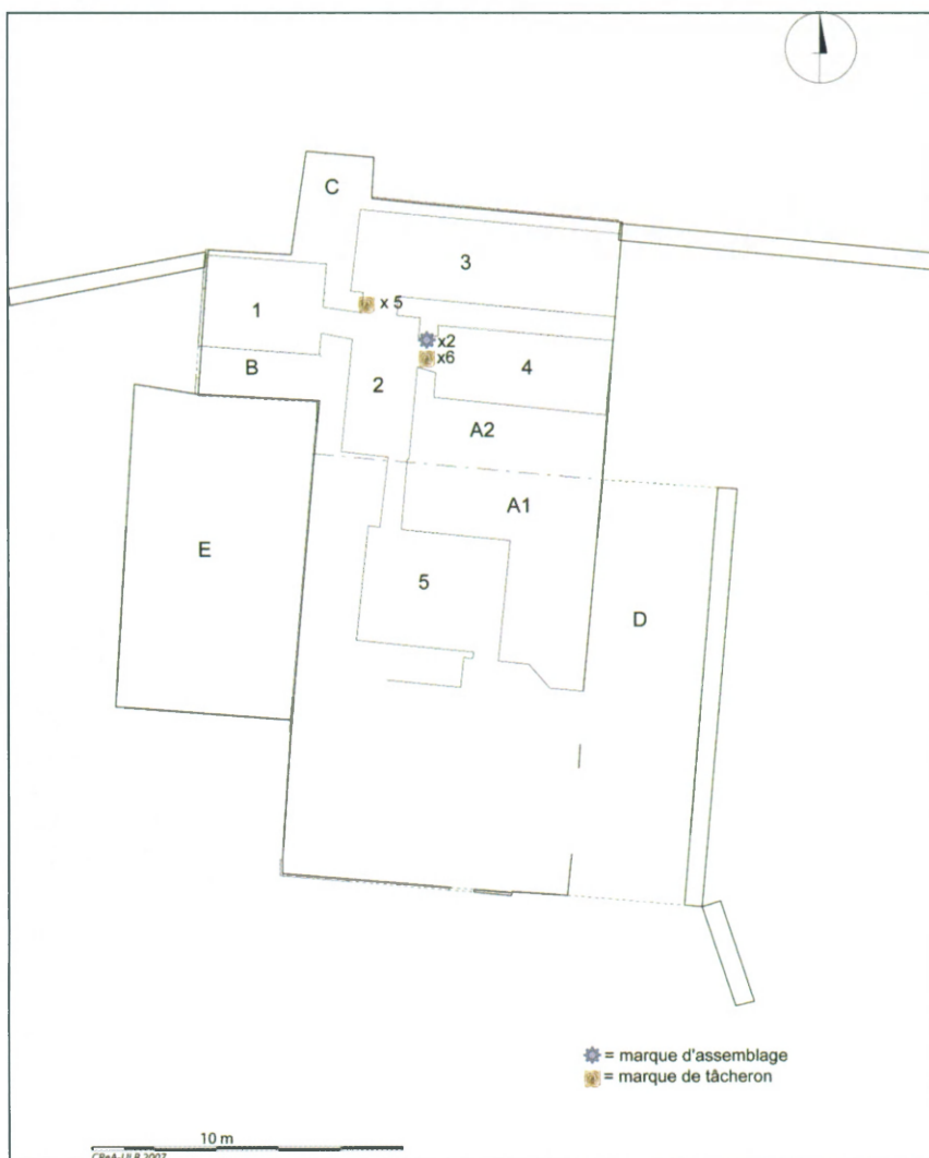
Fig. 4. - Plan d'ensemble du bâtiment au niveau des caves avec répartition des marques. Relevé de l'auteur avec l'aide du CRéA.
