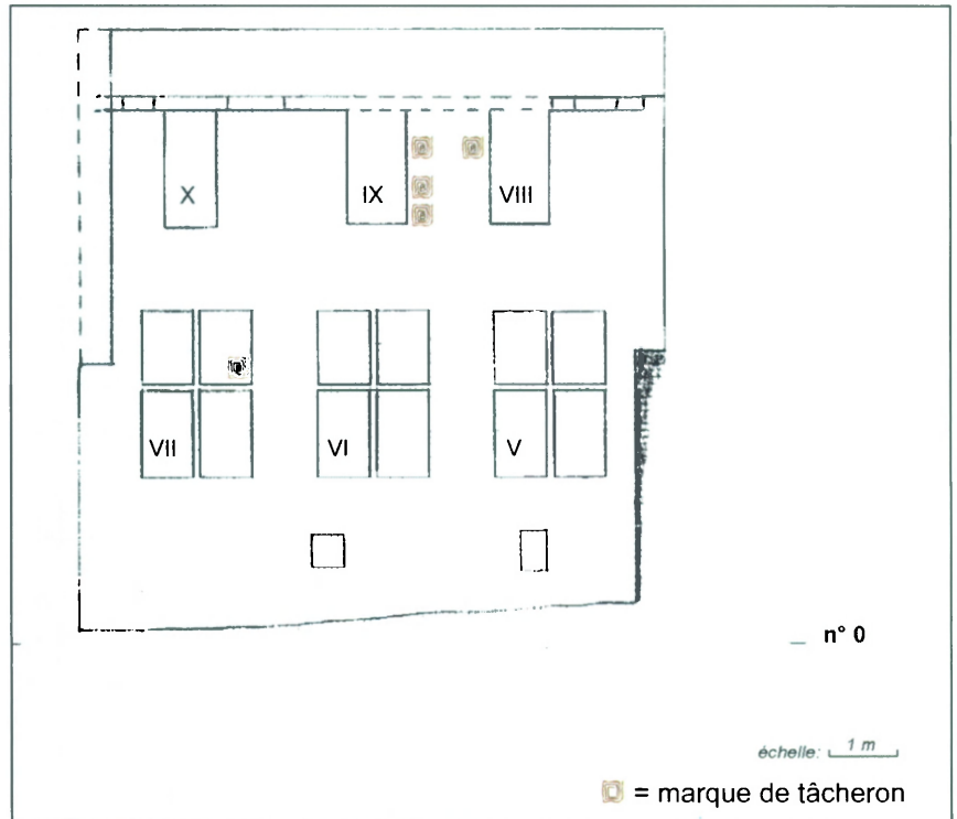
Fig. 16. - Structure A, façade est : schéma d'élévation avec distribution des marques de tâcheron.
