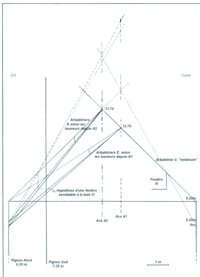
Fig. 32. - Hypothèses de reconstitution de la toiture de la structure A.
