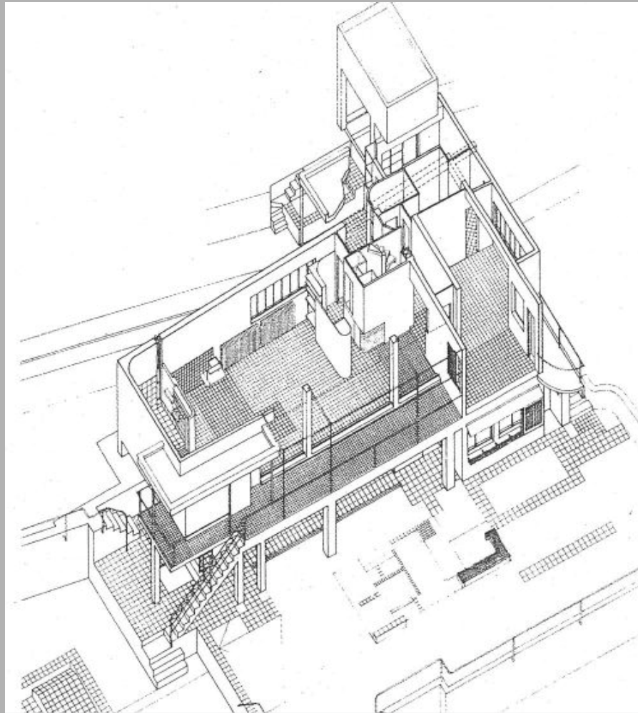
Axonométrie de la Villa, Jean-Paul Rayon, 1969
